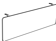
PANEL FRONTOWY Z PŁYTY PET MONTOWANY POD BLATEM BIURKA POJEDYNCZEGO I GABINETOWEGO FRONT PANEL MADE OF PET BOARD MOUNTED UNDER THE TOP OF SINGLE AND EXECUTIVE DESKS L: 102/122*/142*/162 cm D: 1.2 cm H: 38 cm
