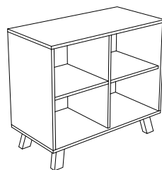
SZAFKA OTWARTA | OPEN CABINET L: 90 cm D: 45 cm H: 80 cm
