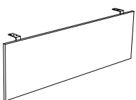
PANEL FRONTOWY Z PŁYTY MEBLOWEJ MONTOWANY POD BLATEM BIURKA POJEDYNCZEGO I GABINETOWEGO FRONT PANEL MADE OF FURNITURE BOARD MOUNTED UNDER THE TOP OF SINGLE AND EXECUTIVE DESKS L: 102/122*/142*/162 cm D: 1.8 cm H: 38 cm
