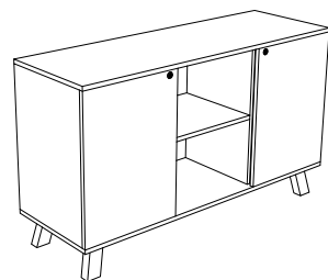
SZAFKA Z PÓLKĄ | CABINET WITH SHELF L: 135 cm D: 45 cm H: 80 cm
